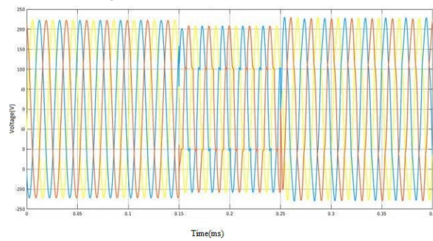
Fig.6.Loadvoltagewithsag
