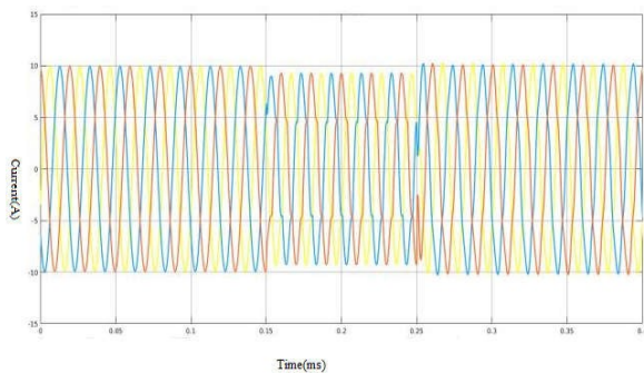
Fig.7.Loadcurrentwithsag
