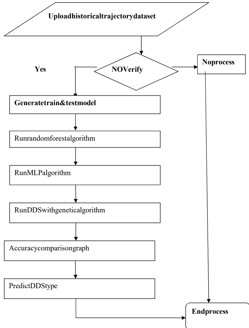
Fig:Dataflowdiagram
